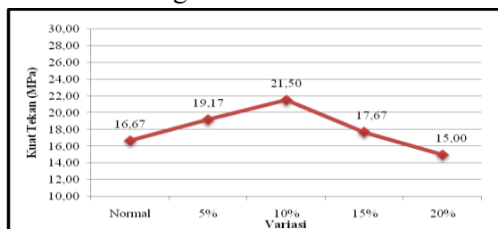
Gambar 4.1. Grafik Kuat Tekan Rata-Rata Umur 7 Hari, Dengan Variasi Abu Sekam Padi Sebesar 0%, 5%, 10%, 15%, 20% Sebagai Substitusi Semen.
