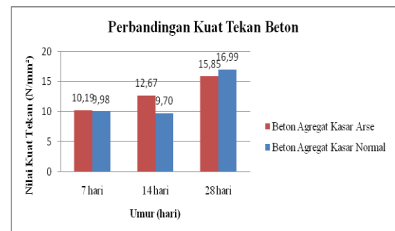
Gambar 2. Diagram Perbandingan Beton Normal dan Beton Arse
