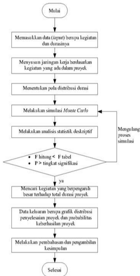
Gambar 2. Bagan Alir Penelitian (sumber: Dokumentasi pribadi)
