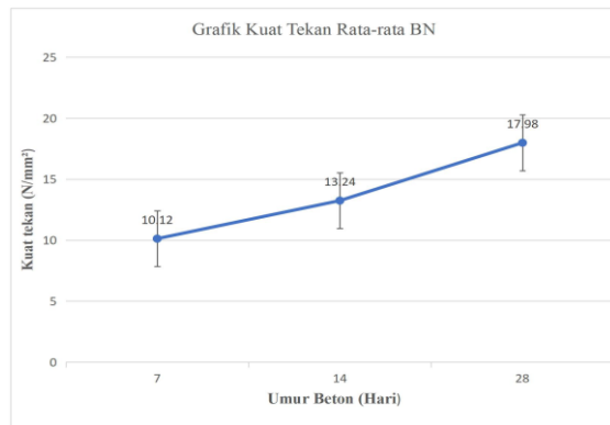
Gambar 1. Grafik Kuat Tekan Rata-Rata Beton Normal Terhadap Umur Beton Tabel 6. Hasil Pengujian Kuat Tekan BV BK 5% dan 5%
