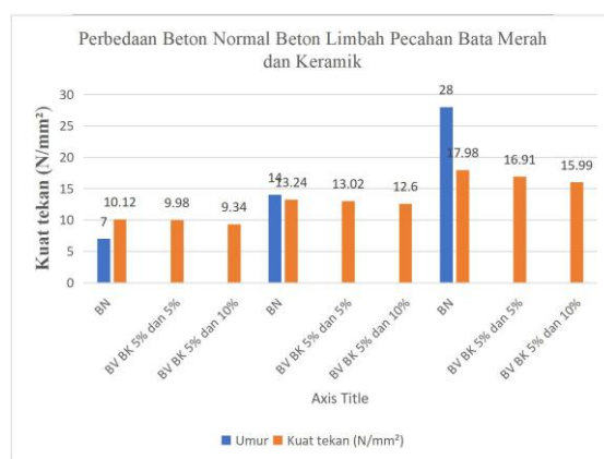
Gambar 4. Perbedaan Nilai Kuat Tekan Beton Gabungan Umur 7, 14 dan 28 Hari
