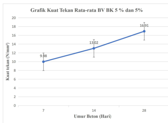
Gambar 2. Kuat tekan rata-rata beton yang dicampur dengan 5% batu bata dan 5% keramik dan penuaan beton Tabel 7. Hasil Pengujian Kuat Tekan BV BK 5% dan 10%
