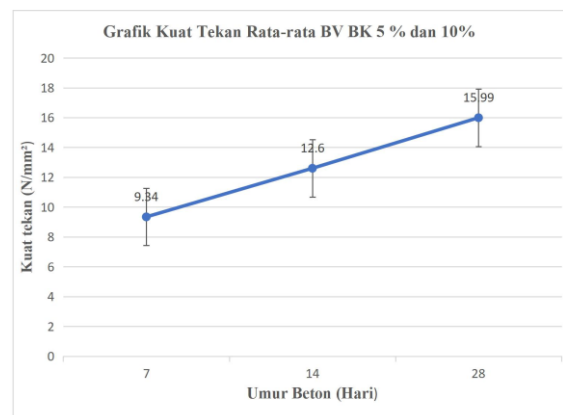
Gambar 3. Grafik Kuat Tekan Rata-Rata Beton Variasi Campuran Bata 5 % Dan 10 % Keramik Terhadap Umur Beton
