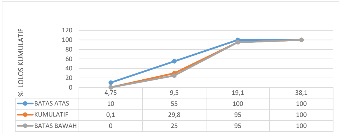
Gambar 4.1 Grafik Hubungan Ukuran Ayakan Dengan Persentase Lolos Ayakan Agregat Kasar (Kerikil)
